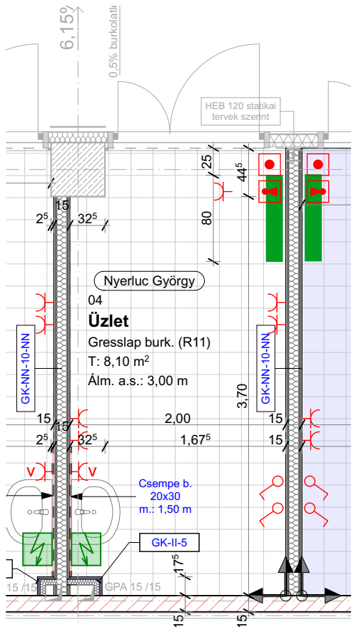
Bérlői földszinti alaprajz
