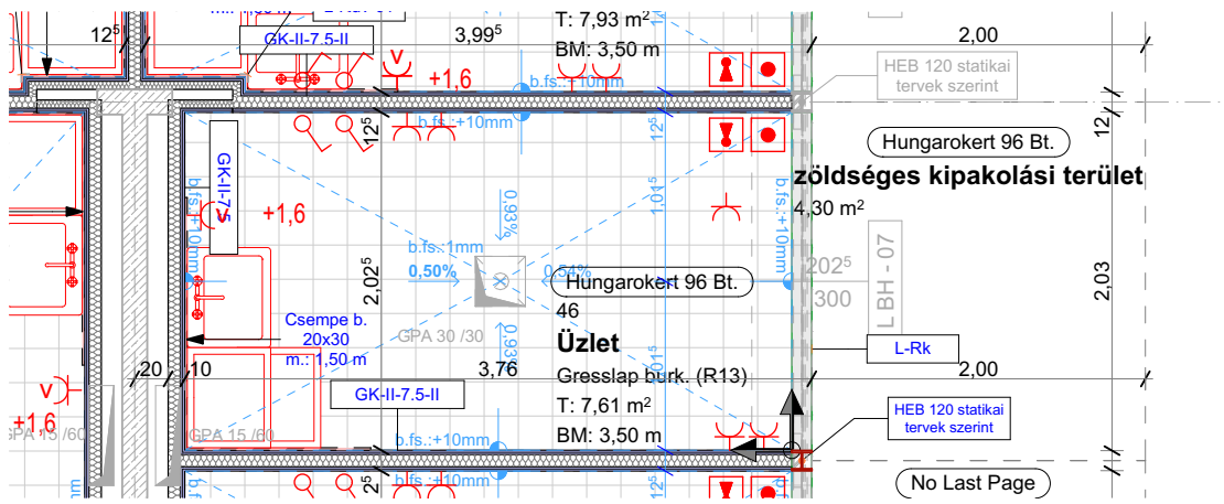
Bérlői földszinti alaprajz
