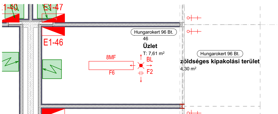
Bérlői állmenyezeti terv
