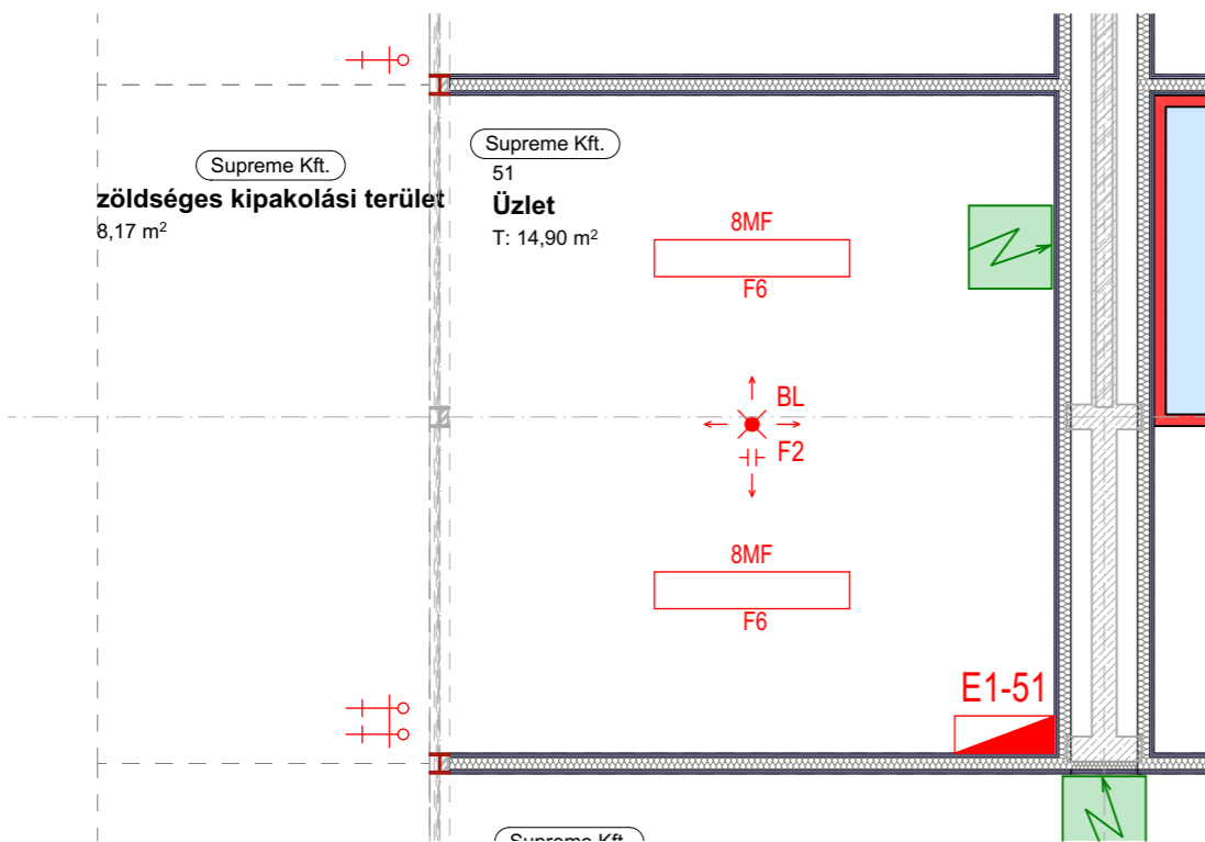
Bérlői állmenyezeti terv
