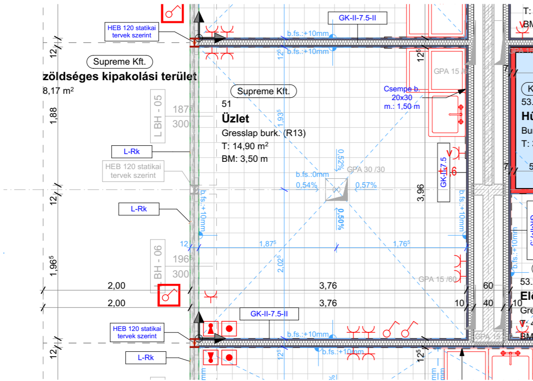
Bérlői földszinti alaprajz
