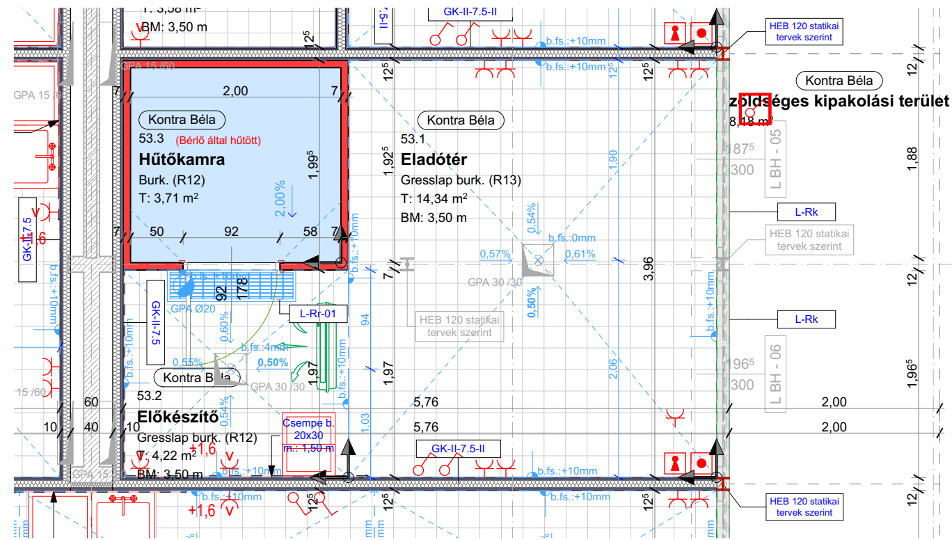
Bérleti földszinti alaprajz
